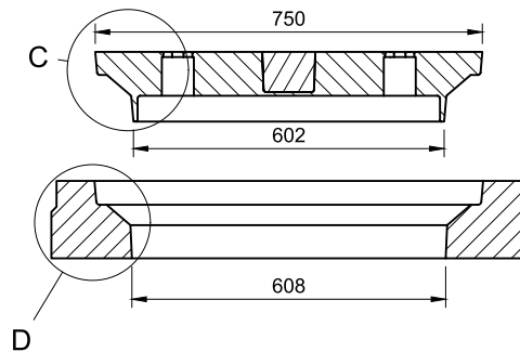
A-A (1:8)
